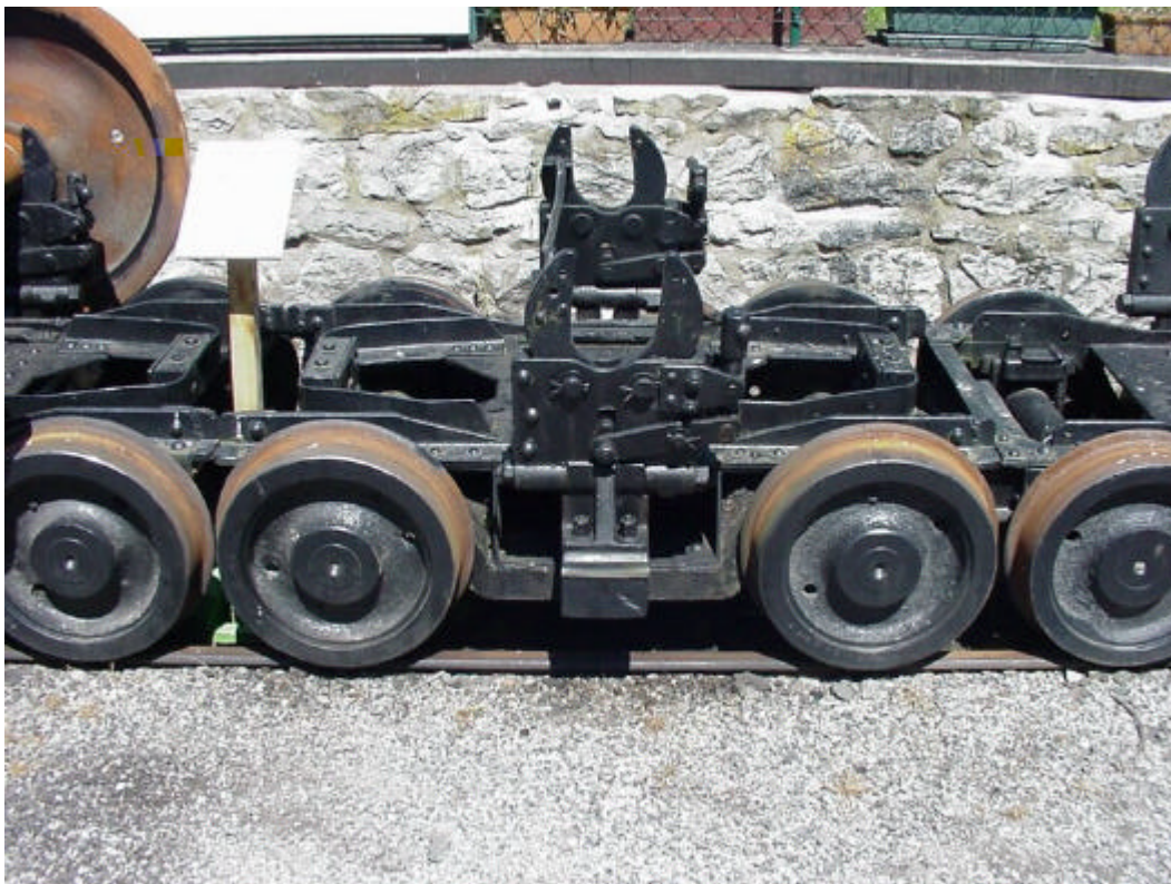
Bild 1: Das Vorbild, HSB Rollbock 99-01-22. Gebaut in 1916 durch die Wagonfabrik Görlitz.
